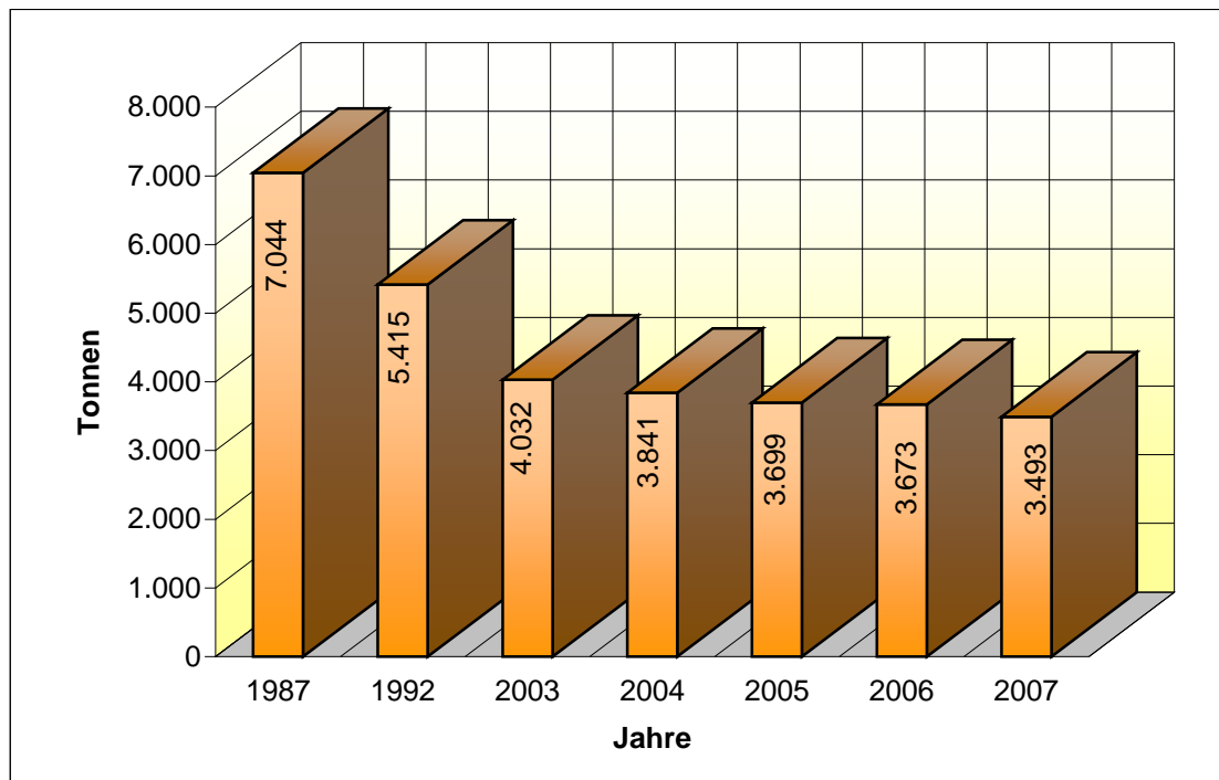
CO 2 – Ausstoß
